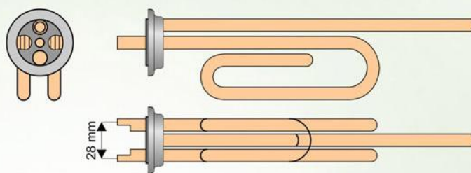
Електронагреватели 2 kW/230V
